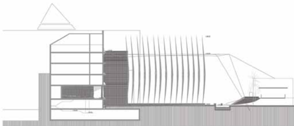
пресек 1-1
