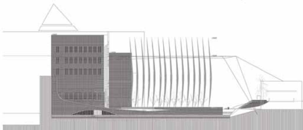
пресек 2-2
